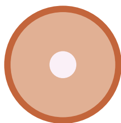
Nella sezione follicolare di un capello liscio c'è un equilibrio di forze
