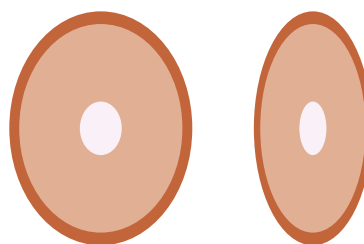
La sezione ellissoidale del follicolo di un capello, oltre che l'aspetto riccio o crespo determina carenza di CMC e punti di debolezza e fragilità
